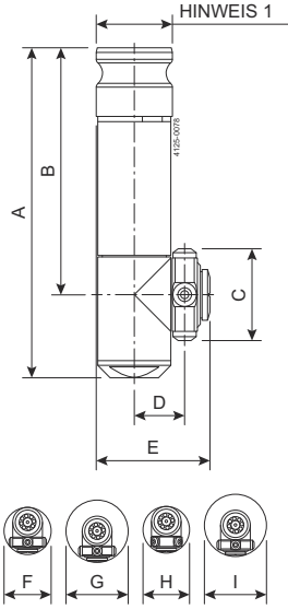
Abbildung 3. Flaches Profil
