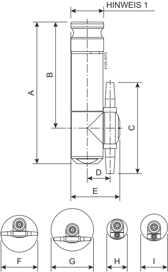
Abbildung 1. 2-Düse
