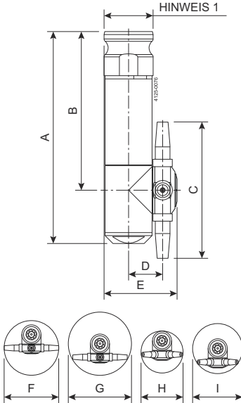
Abbildung 2. 4-Düse
