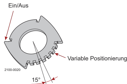
Abbildung 3. Positionierkappe
