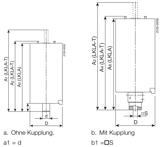
Abbildung 2. Abmessungen - Stelltrieb
