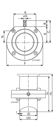
Abbildung 1. Abmessungen - Ventil.
