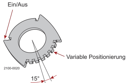
Abbildung 3. Positionierkappe
