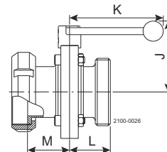
Abbildung 15. LKB mit Gewindestutzen/Mutter und Verschleißschutz
