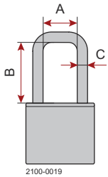
Abbildung 2. Abmessungen - Vorhängeschloss
