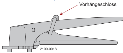
Abbildung 1. Feststellbares Handberteil für stufenlose Einstellung mit Vorhängeschloss
