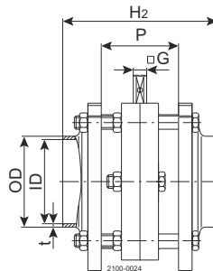
Abbildung 14. c. LKB mit Gewindestutzen/Mutter und Verschleißschutz
