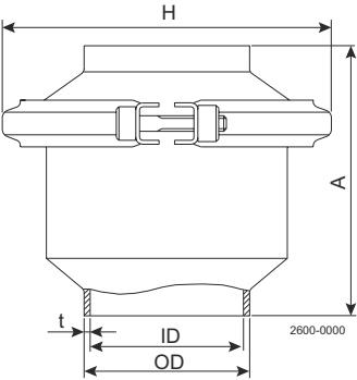
Abbildung 2. Vertikale Montage
