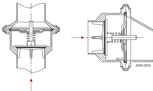
Abbildung 1. Fließrichtung.
