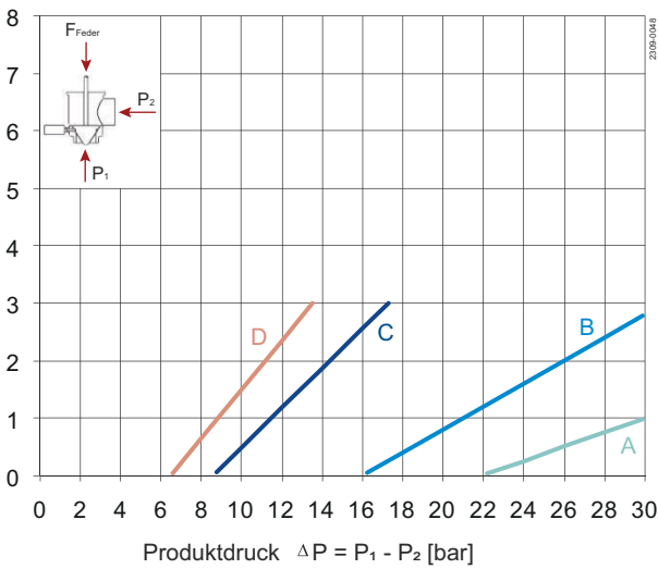
Abbildung 3. ø89 Stelltrieb
