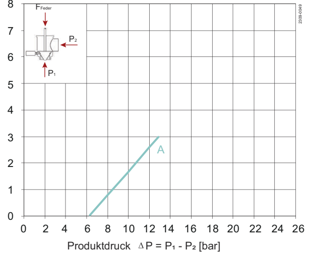
Abbildung 6. ø199 Stelltrieb
