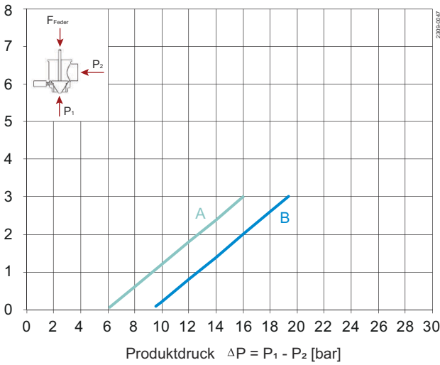
Abbildung 3. ø89 Stelltrieb
