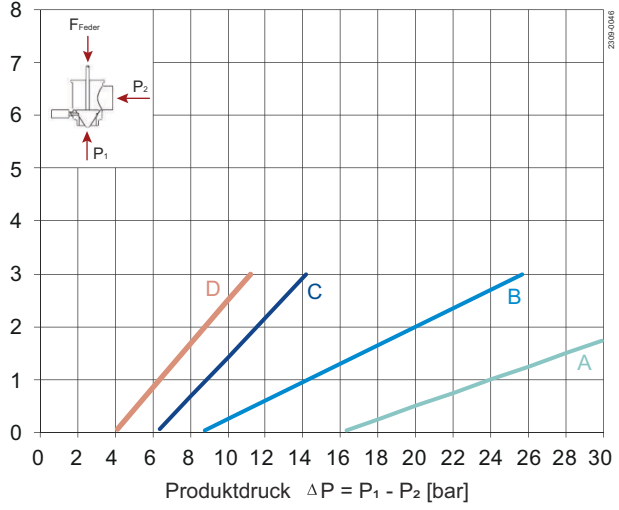
Abbildung 4. ø133 Stelltrieb mit Standardfeder
