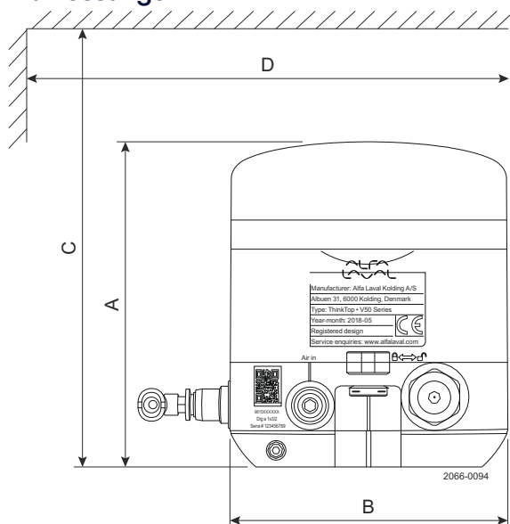
Abbildung 1. ThinkTop V 50
