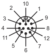
M12-Option (12-poliger A-codierter Stecker)
