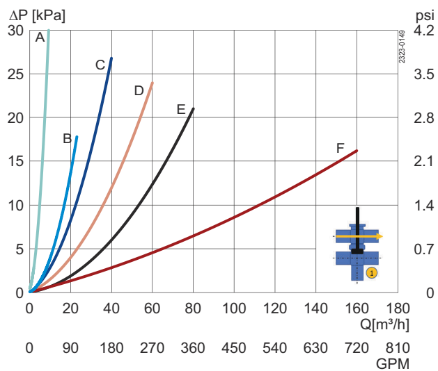
Abbildung 1. Druckabfall-/Leistungsdiagramm, oberes Gehäuse
