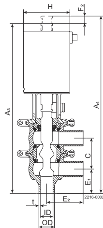
Abbildung 2. Umschaltventil
