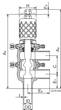
Abbildung 4. Manuelles Umschaltventil
