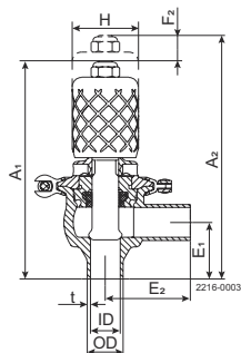
Abbildung 3. Manuelles Absperrventil
