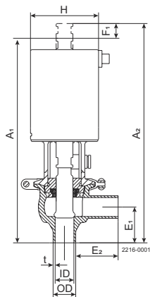
Abbildung 1. Absperrventil
