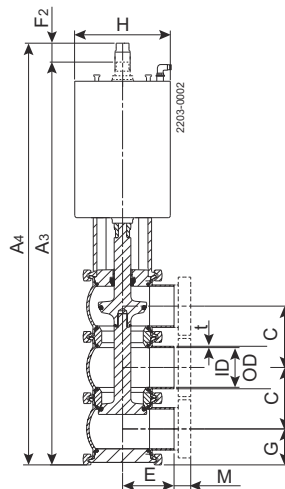
Abbildung 2. Umschaltventil
