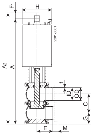
Abbildung 1. Absperrventil
